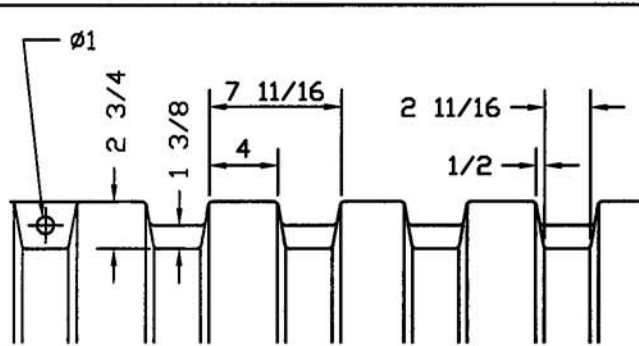
RIB DIMENSIONS 1/8 SCALE
